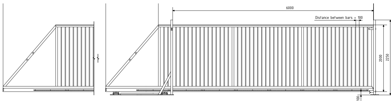
ODEN Exempelritning 6 x 2 m
